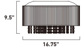
E23133-10PC Flush Mount
