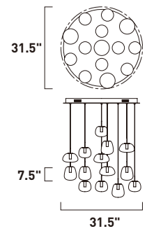
E21129-11WT Pendant
