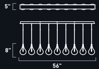
E23119-18 Pendant
