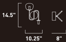
E21123-11WT Wall Mount
