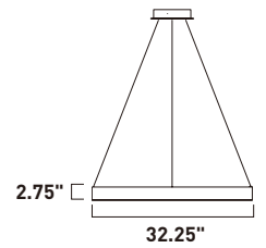
E24297-AL, -COF, -SC Pendant
