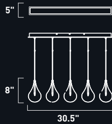
E23115-18 Pendant
