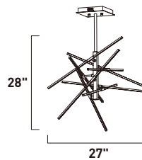
E20695-PC Pendant
