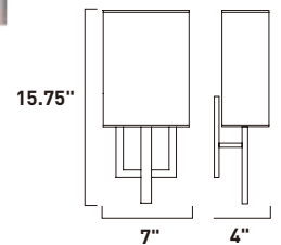
E21082-01SN Wall Mount
