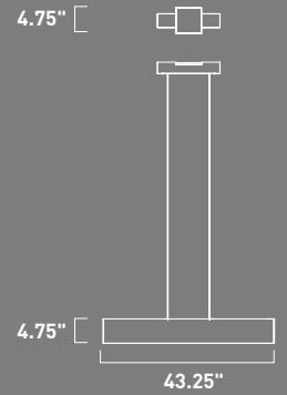
E22904-BZ Pendant
