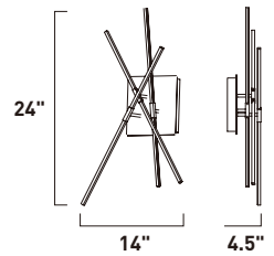
E20691-PC Wall Mount
