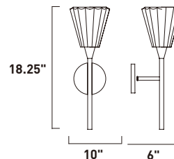
E20191-19 Wall Mount
