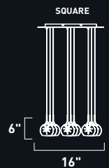
E20106-24, -25 Pendant
