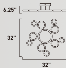
E21146-01PC Semi-Flushmount
