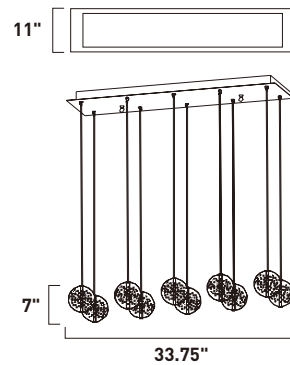
E24256-91PC Pendant
