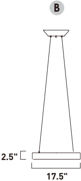
E20225-MW Pendant
