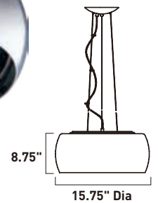
E21205-10PC Pendant
