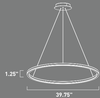
E22845-MW Pendant
