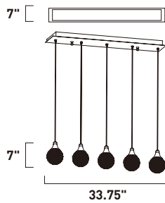
E24025-20PC Pendant
