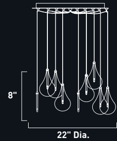
E20115-18 Pendant
