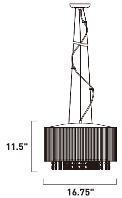
E23135-10PC Pendant
