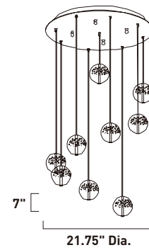
E24254-91PC Pendant
