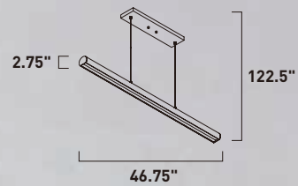
E41467-SA, WT Pendant A
