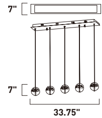
E24257-91PC Pendant
